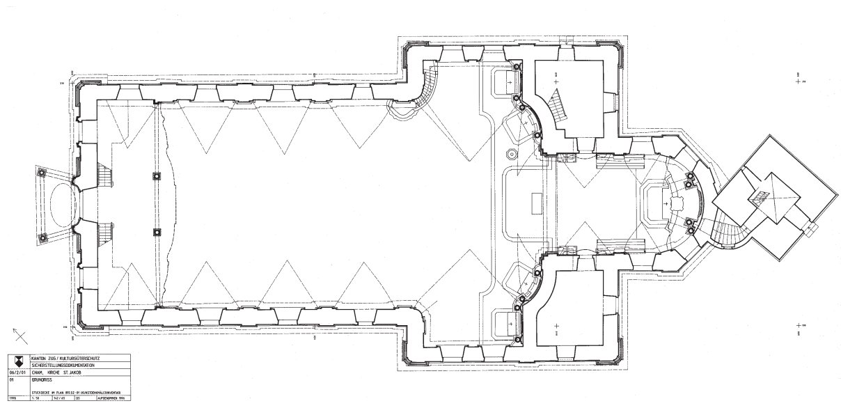
B Piano di costruzione (pianta); rappresentazione molto ridotta (scala originale 1:50).
