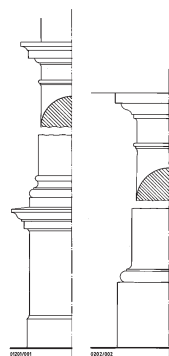
E1 Piano di dettaglio di elementi architettonici e decorativi (vedute/profili); rappresentazione ridotta (scala originale 1:5).
